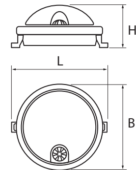
Рис.1 Светильник PBH-PC3-RSI SENSOR
