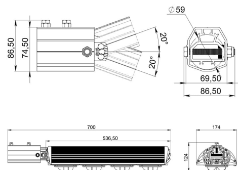
Габаритный чертёж
