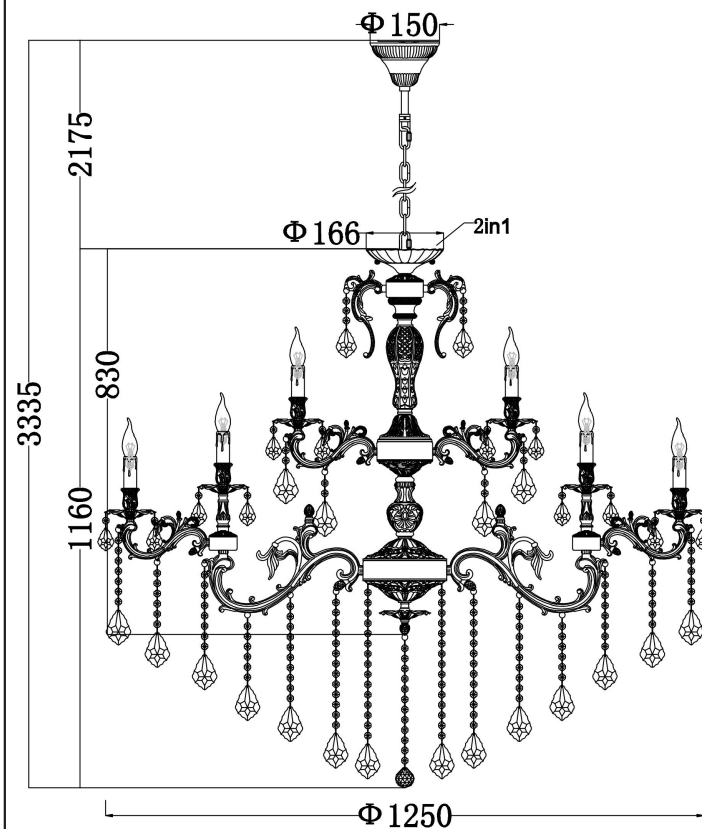
DIA882-PL-30-G 尺寸图
