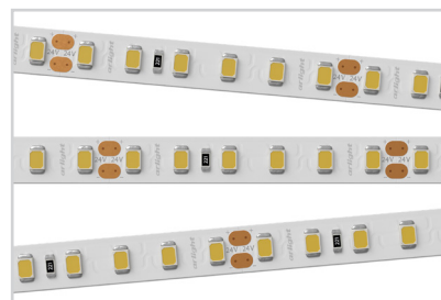
020393(B) RT 2-5000 24V Warm3000 2x
