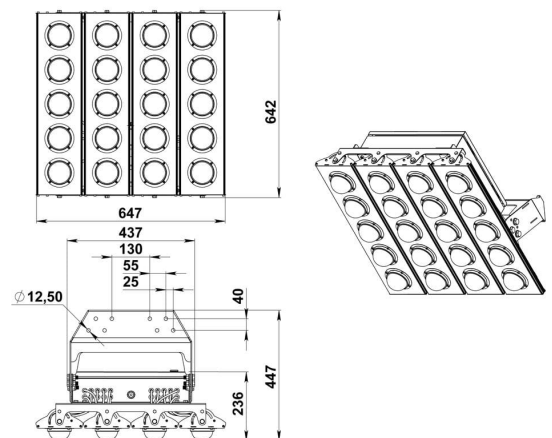
Габаритный чертёж
