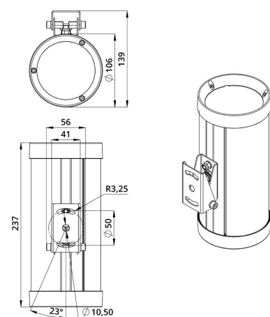
Габаритный чертеж
