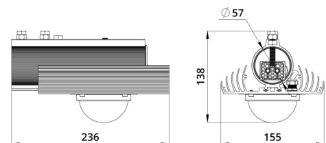
Габаритный чертеж
