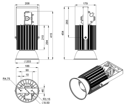
Габаритный чертеж
