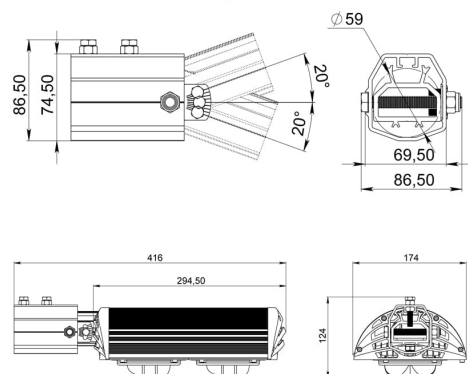
Габаритный чертёж
