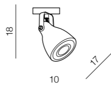
Bremen wall AZ2370 GU10 1x MAX 40W concrete/metal
