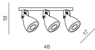
Bremen 3 AZ2371 GU10 3x MAX 40W concrete/metal
