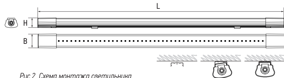
Рис.2 Схема монтажа светильника
